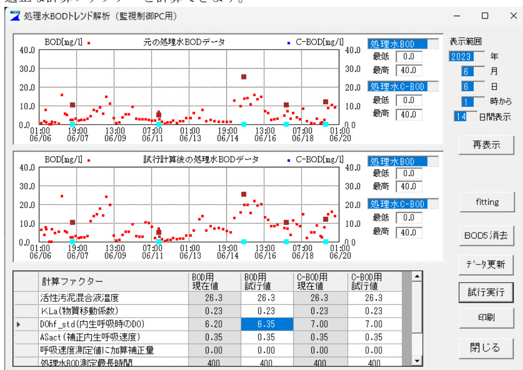
図の●は TSA-5 測定値、■は公定法の BOD 値、BOD 用試行値欄の設定値を変えて繰り返し計算することで、適正な DOhf_std を設定できます。[fitting]をクリックすると自動で適正な計算ファクターを計算できます。
