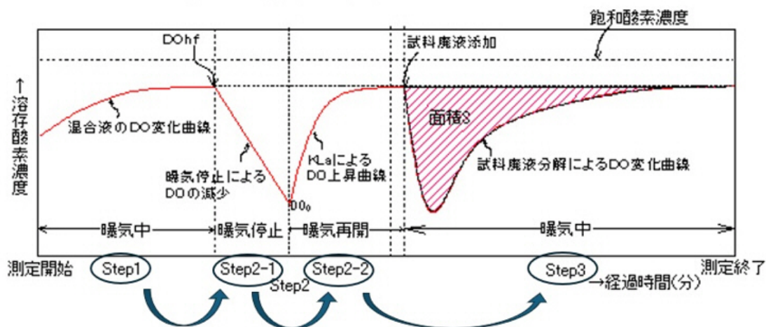
図1-1:DO変化の基本パターン
