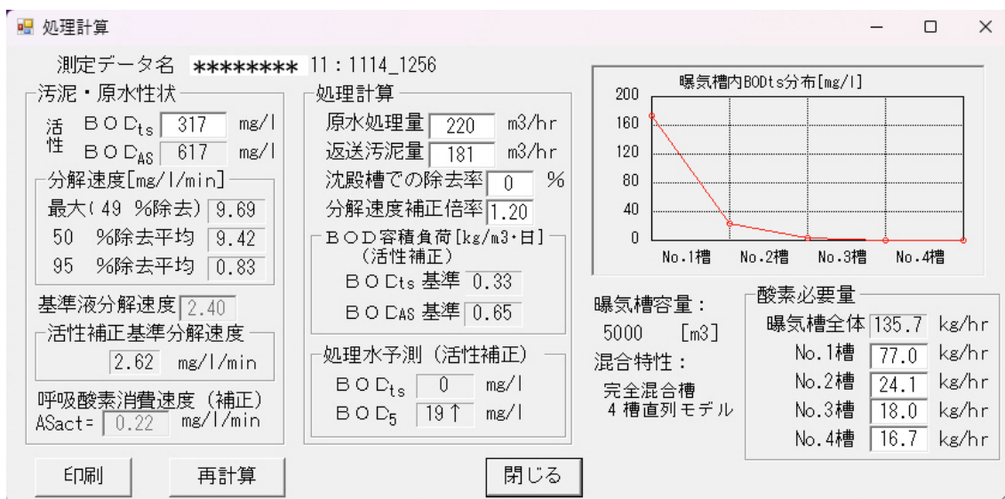
図 4-2-3：処理計算（連続式活性汚泥）
